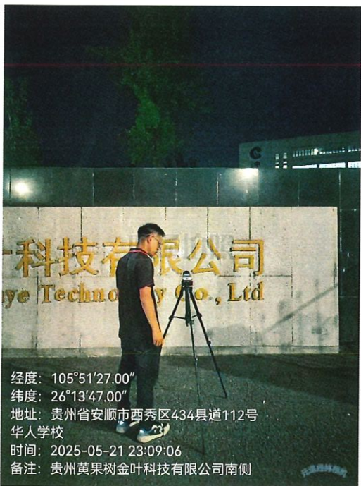
厂界南侧噪声检测图片（夜间）
